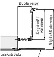
Dimension Ablauf-Steigrohr
